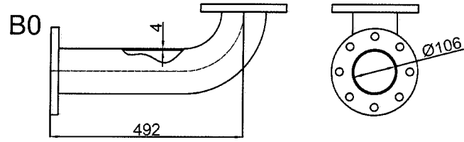
Rys.6 Zasilanie - wstepny_element
