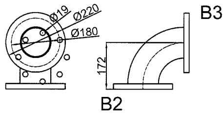
Rys.8 zasilanie - 3_segment_kolanko
