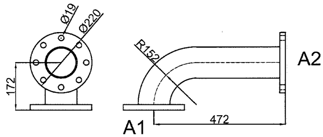
Rys.2 Powrót - 2_segment
