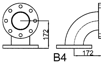
Rys.9 zasilanie - koncowe_kolanko
