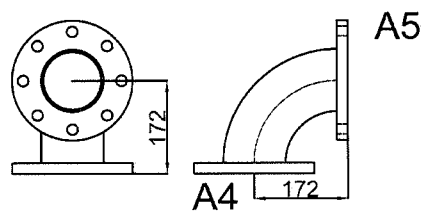
Rys.5 Powrót - końcowe_kolanko
